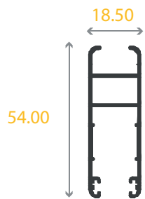
3416 Hoja
