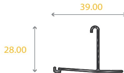
3639 Adaptador de Marco
