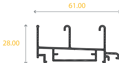
3641 Marco de Ventana
