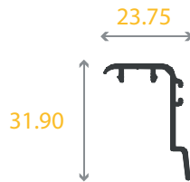
3417 Entrecierre
